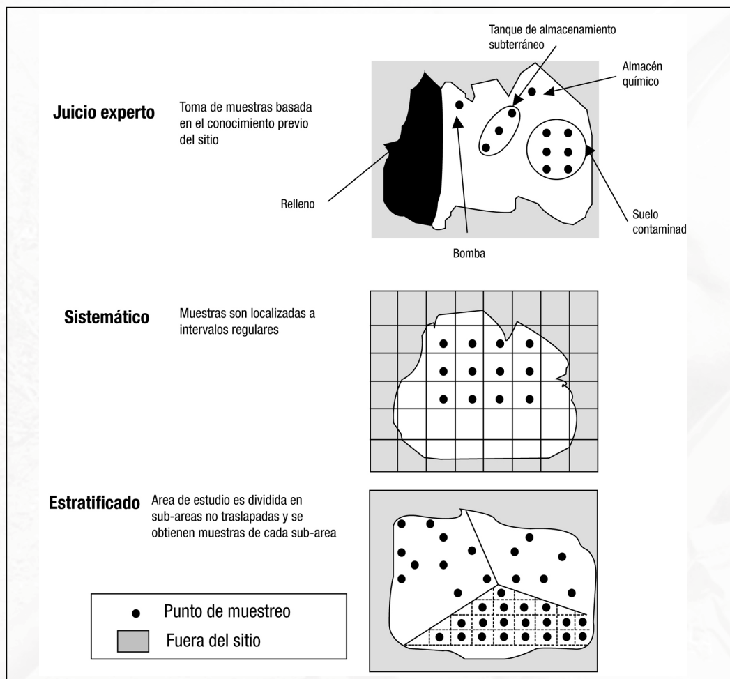
Figura 5: Patrones de muestreo considerados por la Guía Neozelandesa para el muestreo de suelo/sitios contaminados.
